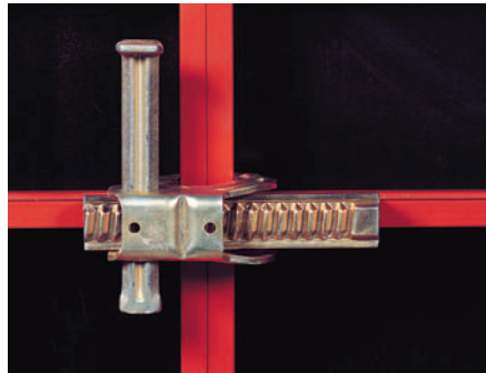
Soit au niveau de la jonction d'éléments standards...
