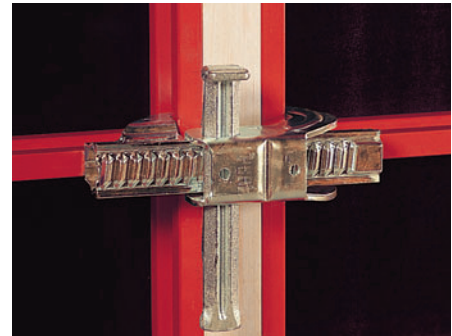
...soit avec des cales bois jusqu'à une épaisseur de 12 cm.
